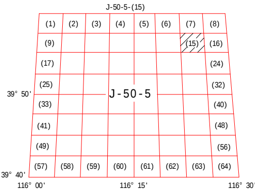
图 J. 3. 2—1 1 : 10000 地形图国际分幅编号
