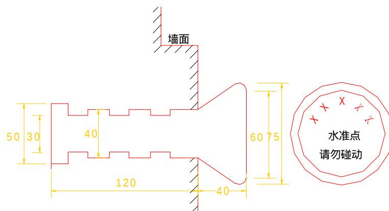
图 G.2.3 墙脚水准标志埋设
