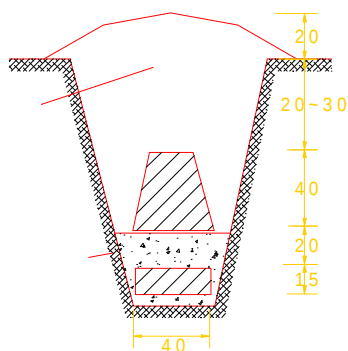
图 C.2.1 各等平面控制点标石埋设（单位：cm）
