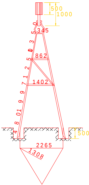
图 B. 1. 1 4. 5m 钢寻常标觐标 (单位: mm)
