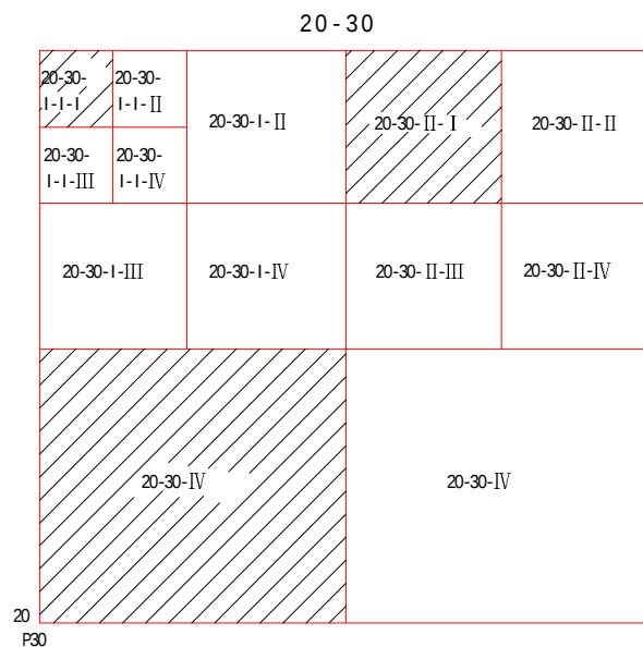
图 J. 1. 2 正方形分幅编号
