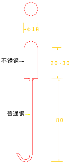
图 G.1.2 不锈钢标志 (单位:mm)
