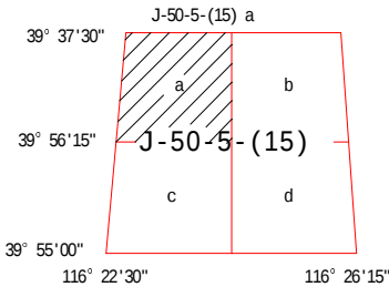
图 J. 3. 2—2 1 : 5000 地形图国际分幅编号
