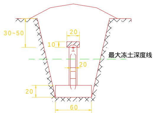
图 G.2.4 混凝土柱普通水准标石埋设
