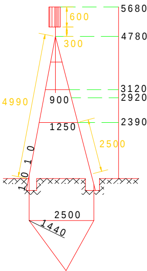
图 B. 1. 2 木质寻常标觐标 (单位: mm)
