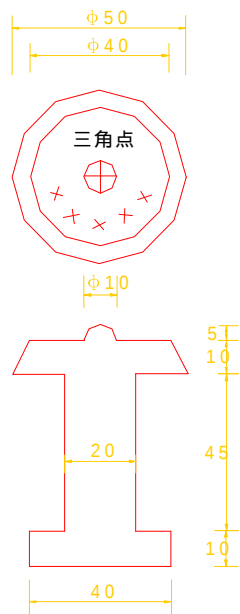
图 C.1.1 金属标志 (单位: mm)
